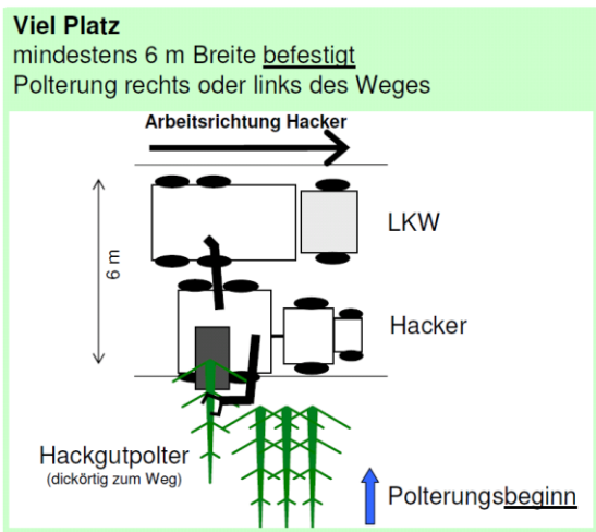
Abb. 1+2: Holzbereitstellung Waldhackholz
